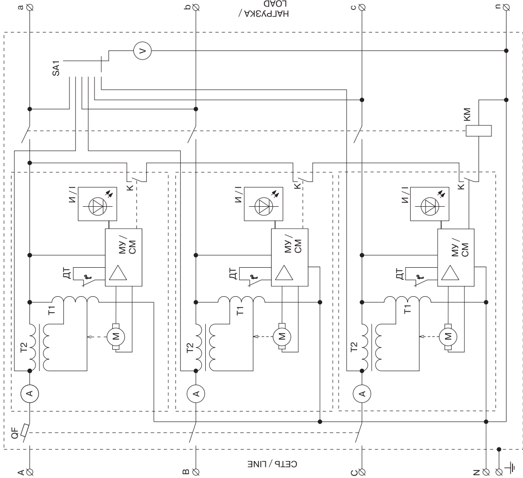
Рисунок 4 б – Структурные схемы стабилизаторов: СНИЗ-15 кВА; СНИЗ-20 кВА; СНИЗ-30 кВА; СНИЗ-45 кВА; СНИЗ-60 кВА с дополнительным вольтдобавочным трансформатором
